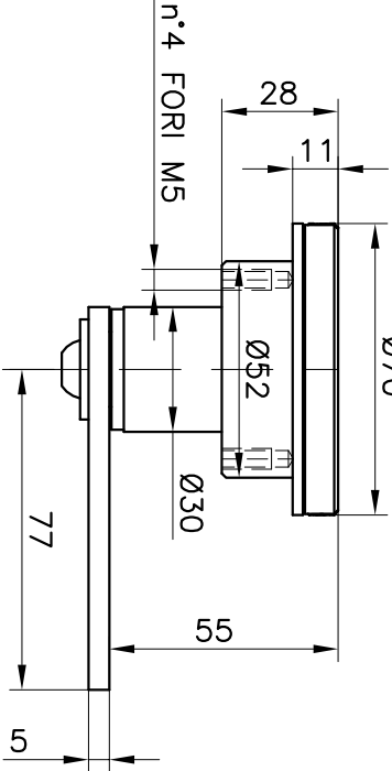
CHIUSURA COD.102010400 Closing
