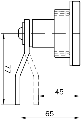
CHIUSURA COD.102010600 Closing
