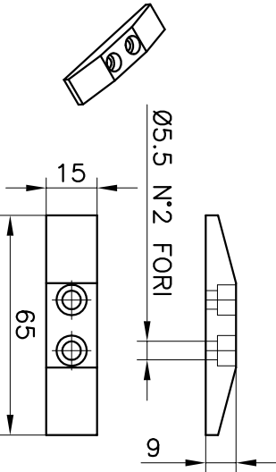
TACCHETTO COD.129011500 Cleat
