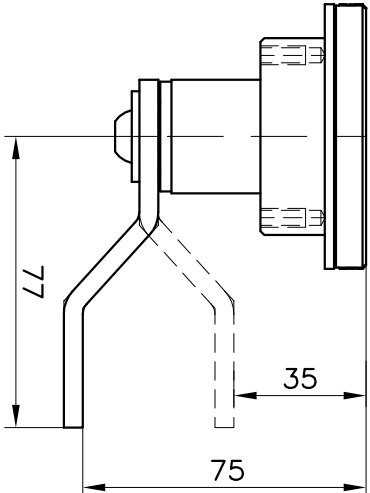
MATERIALE: ACCIAIO INOX AISI 316 Material: Stainless steel aisi 316
