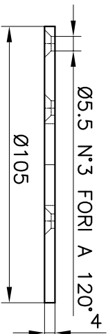
MATERIALE: ACCIAIO INOX AISI 316 Material: Stainless steel aisi 316
