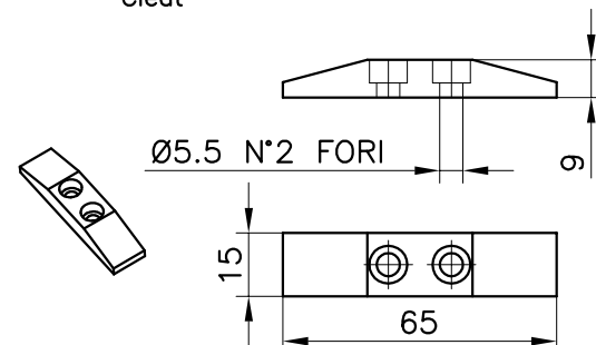
TACCHETTO COD.129011500 Cleat
