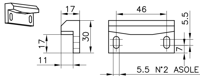
TACCHETTO COD.129011600 Cleat
