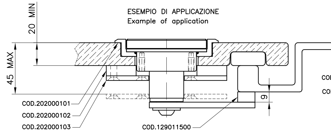
TACCHETTO COD.129011500 Cleat
