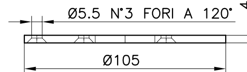
FLANGIA DI FISSAGGIO COD.202000103 Fixing plate
