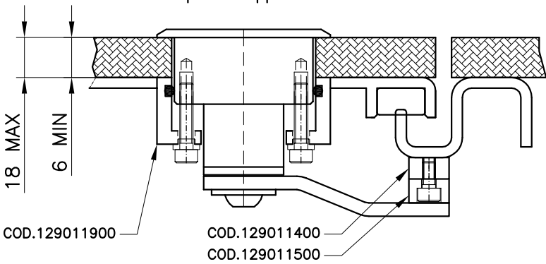
ESEMPIO DI APPLICAZIONE Example of application
