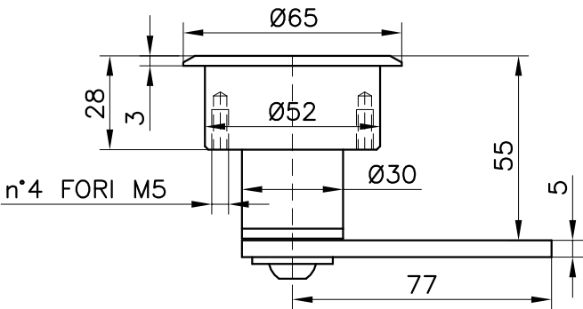
CHIUSURA COD.102060500 Closing
