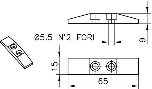
TACCHETTO COD.129011500 Cleat
