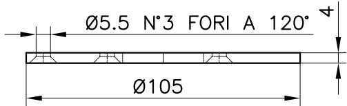
FLANGIA DI FISSAGGIO COD.202000103 Fixing plate
