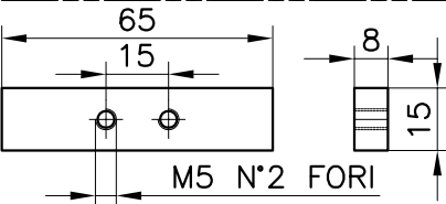
TACCHETTO ACCIAIO INOX AISI 316 COD.129011700 Stainless steel AISI 316 cleat
