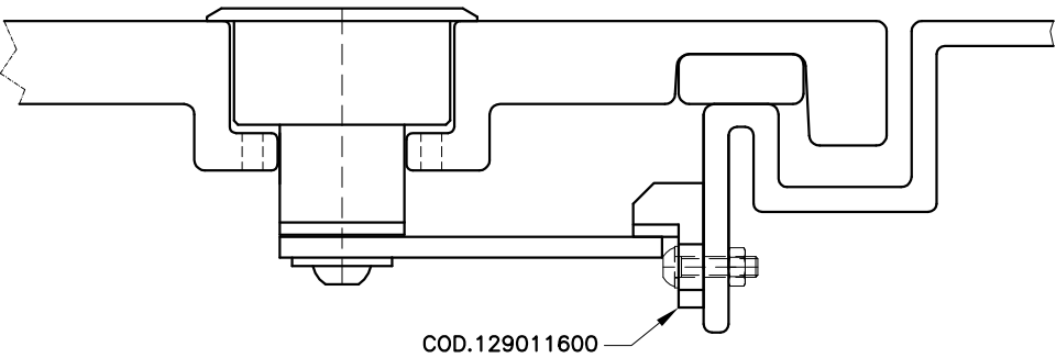
TACCHETTO COD.129011600 Cleat
