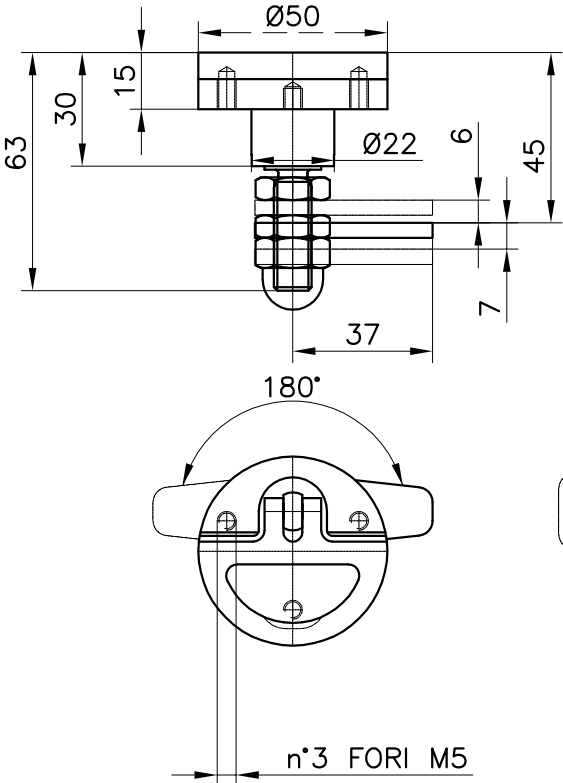
CHIUSURA COD.102100400 Closing
