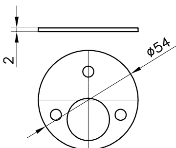
FLANGIA DI FISSAGGIO COD.202010016 Fixing plate
