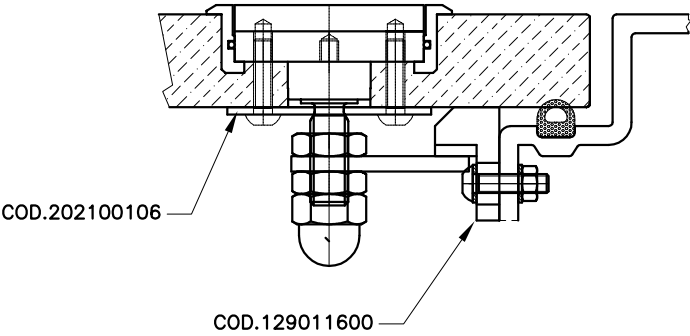
TACCHETTO COD.129011600 Cleat
