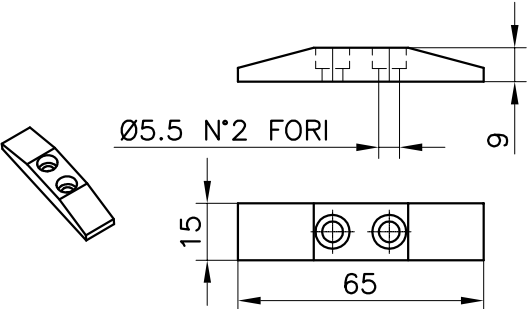
TACCHETTO COD.129011500 Cleat
