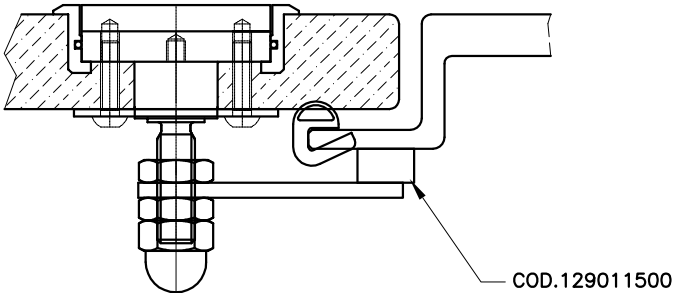
ESEMPIO DI APPLICAZIONE Example of application
