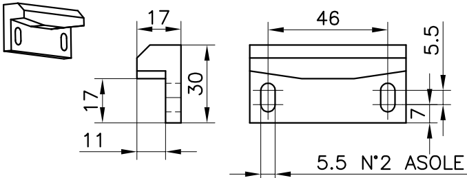
TACCHETTO COD.129011600 Cleat
