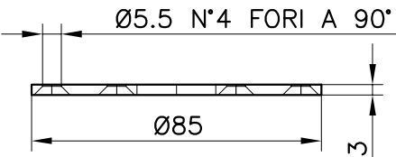
FLANGIA DI FISSAGGIO COD.202100108 Fixing plate
