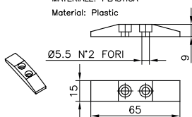
TACCHETTO COD.129011500 Cleat MATERIALE: PLASTICA Material: Plastic
