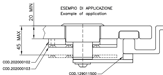
TACCHETTO COD.129011500 Cleat MATERIALE: PLASTICA Material: Plastic
