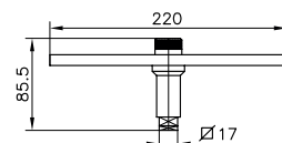
MATERIALE: ACCIAIO INOX AISI 316 Material: Stainless steel AISI 316
