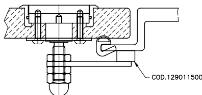
ESEMPIO DI APPLICAZIONE Example of application
