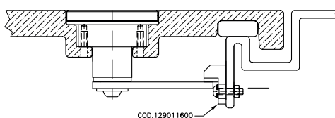
TACCHETTO COD.129011600 Cleat MATERIALE: PLASTICA Material: Plastic
