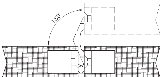
ESEMPIO DI APPLICAZIONE EXAMPLE OF APPLICATION
