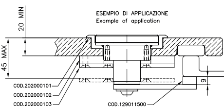
TACCHETTO COD.129011500 Cleat MATERIALE: PLASTICA Material: Plastic
