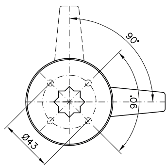
ESEMPIO DI APPLICAZIONE Example of application
