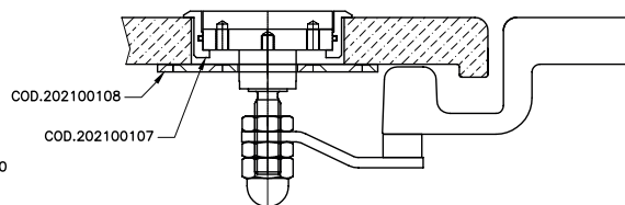
ESEMPIO DI APPLICAZIONE Example of application
