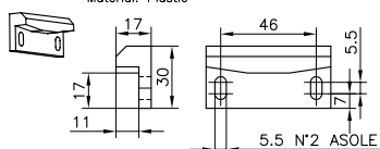
TACCHETTO COD.129011600 Cleat MATERIALE: PLASTICA Material: Plastic
