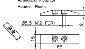
TACCHETTO COD.129011500 Cleat MATERIALE: PLASTICA Material: Plastic
