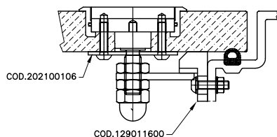
ESEMPIO DI APPLICAZIONE Example of application
