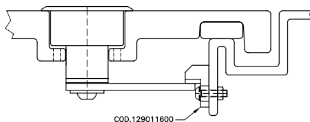
ESEMPIO DI APPLICAZIONE Example of application
