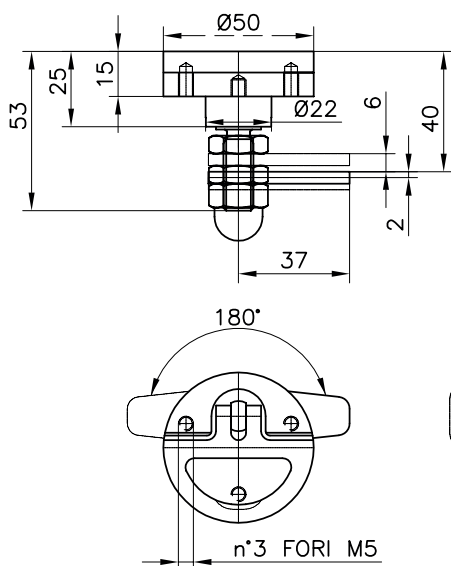
ESEMPIO DI APPLICAZIONE Example of application
