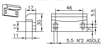
TACCHETTO COD.129011600 Cleat MATERIALE: PLASTICA Material: Plastic
