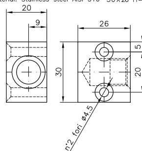
RISCONTRO cod. 215020106
