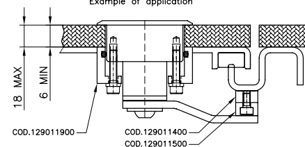
ESEMPIO DI APPLICAZIONE Example of application
