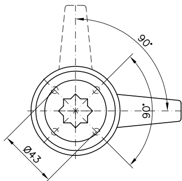
ESEMPIO DI APPLICAZIONE Example of application
