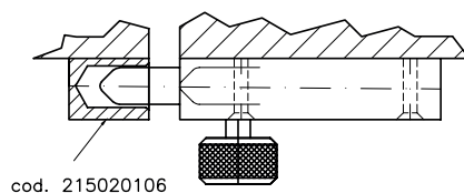
RISCONTRO cod. 215020106
