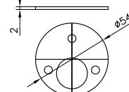
FLANGIA DI FISSAGGIO COD.202100106 Fixing plate MATERIALE: ACCIAIO INOX AISI 316 Material: Stainless steel aisi 316
