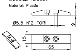
TACCHETTO COD.129011500 Cleat MATERIALE: PLASTICA Material: Plastic
