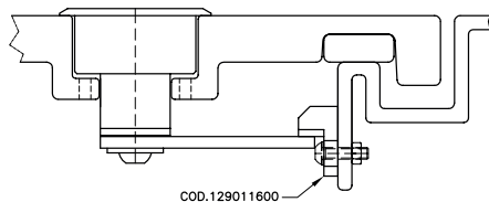
ESEMPIO DI APPLICAZIONE Example of application
